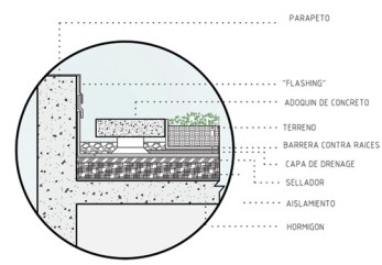
DETALLE DE TECHO VERDE ESCALA: 12" = 1'-0"
