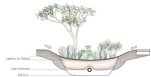
DETALLE DE JARDIN DE LLUVIA ESCALA: 12" = 1'-0"
