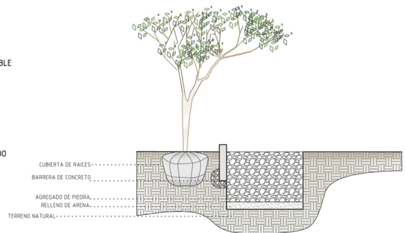
DETALLE DE ZANJA DE FILTRACION ESCALA: 12" = 1'-0"
