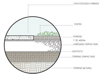
DETALLE DE PAVIMENTO ESCALA: 12" = 1'-0"
